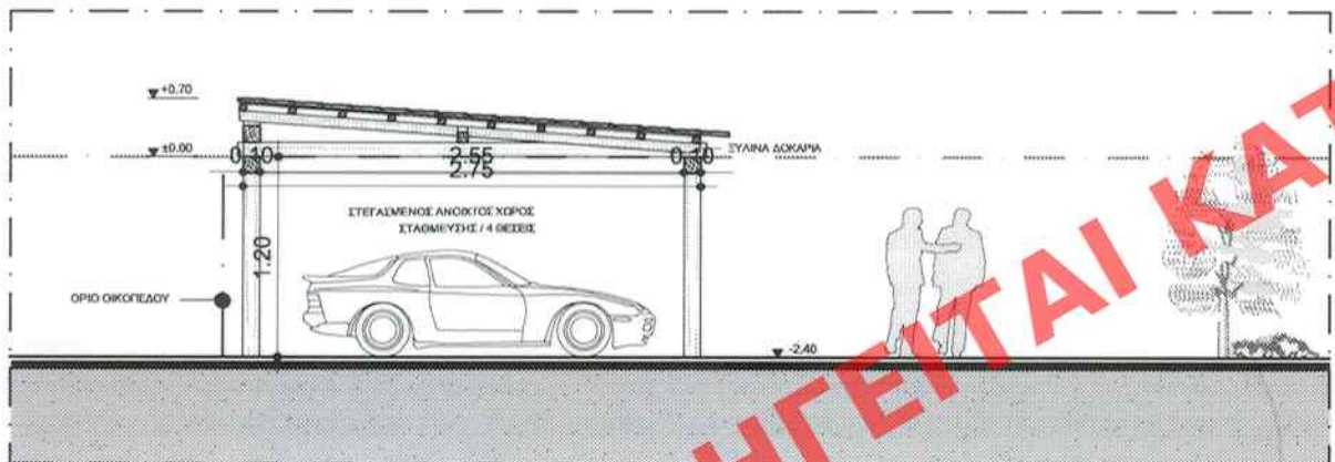
ΤΟΜΗ Α-Α, ΚΛ. 1:50
